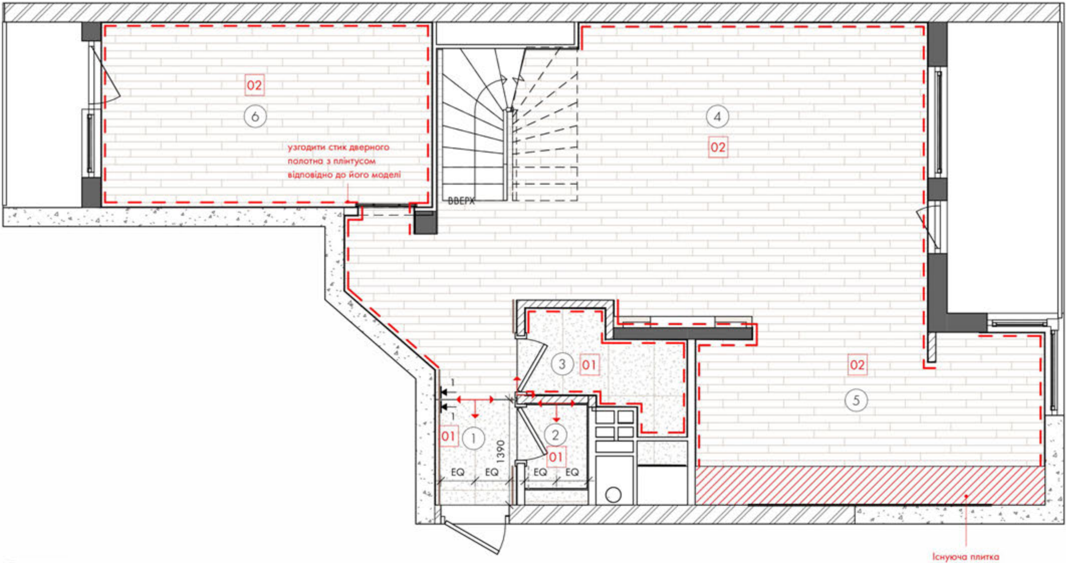
План підлог 1 : 50
