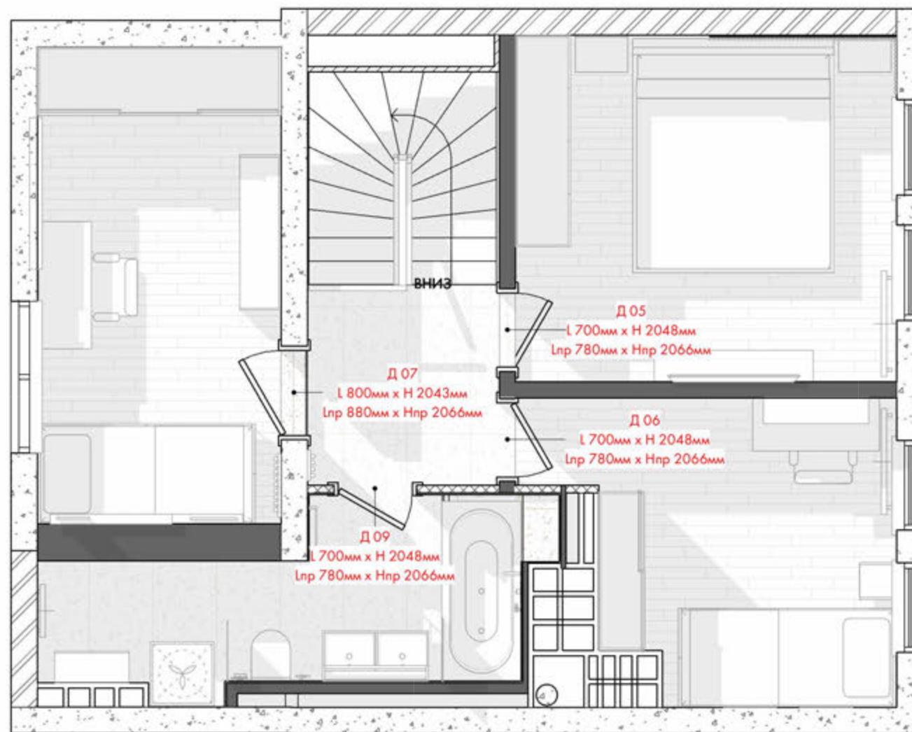
План заповнення дверних прорізів 2 поверх
