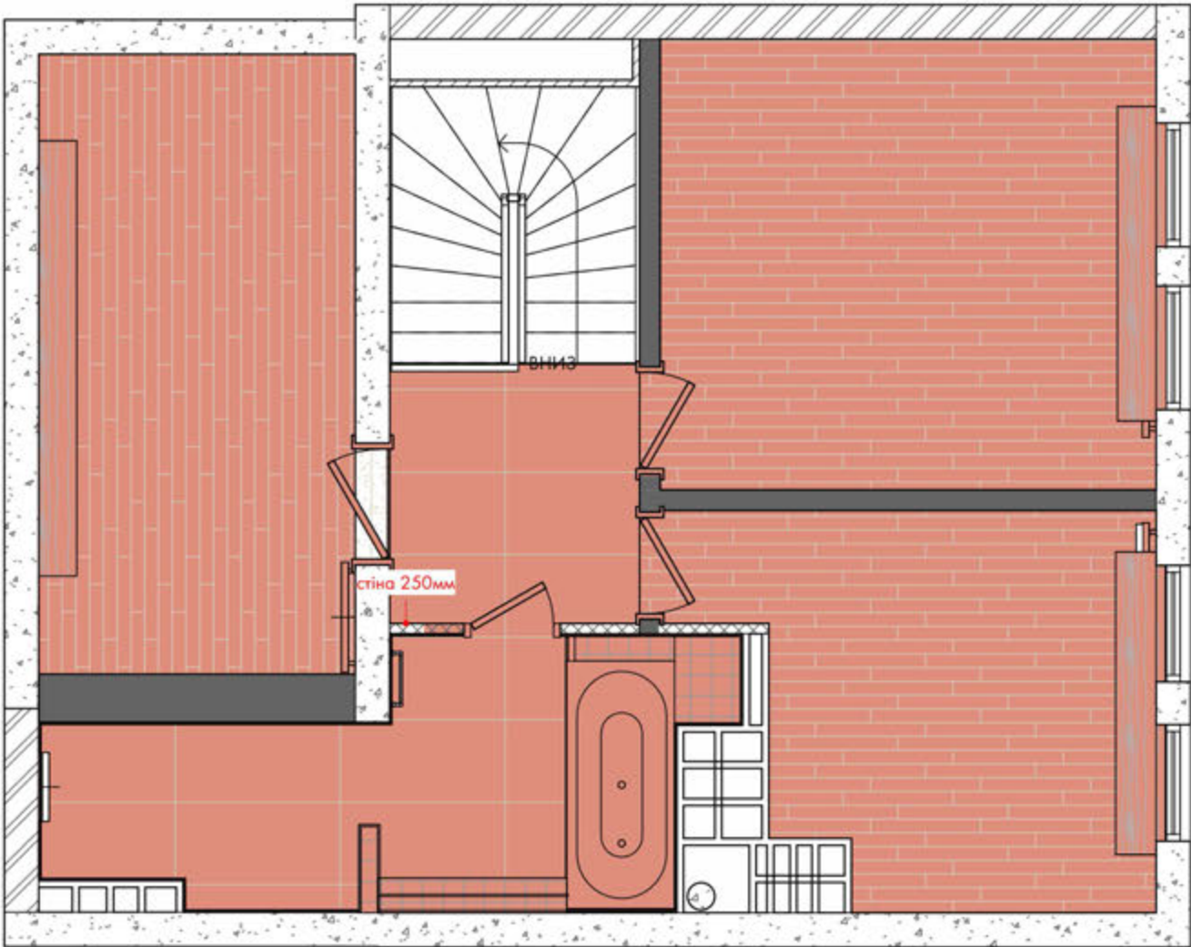
План демонтажу 2 поверх 1 : 50
