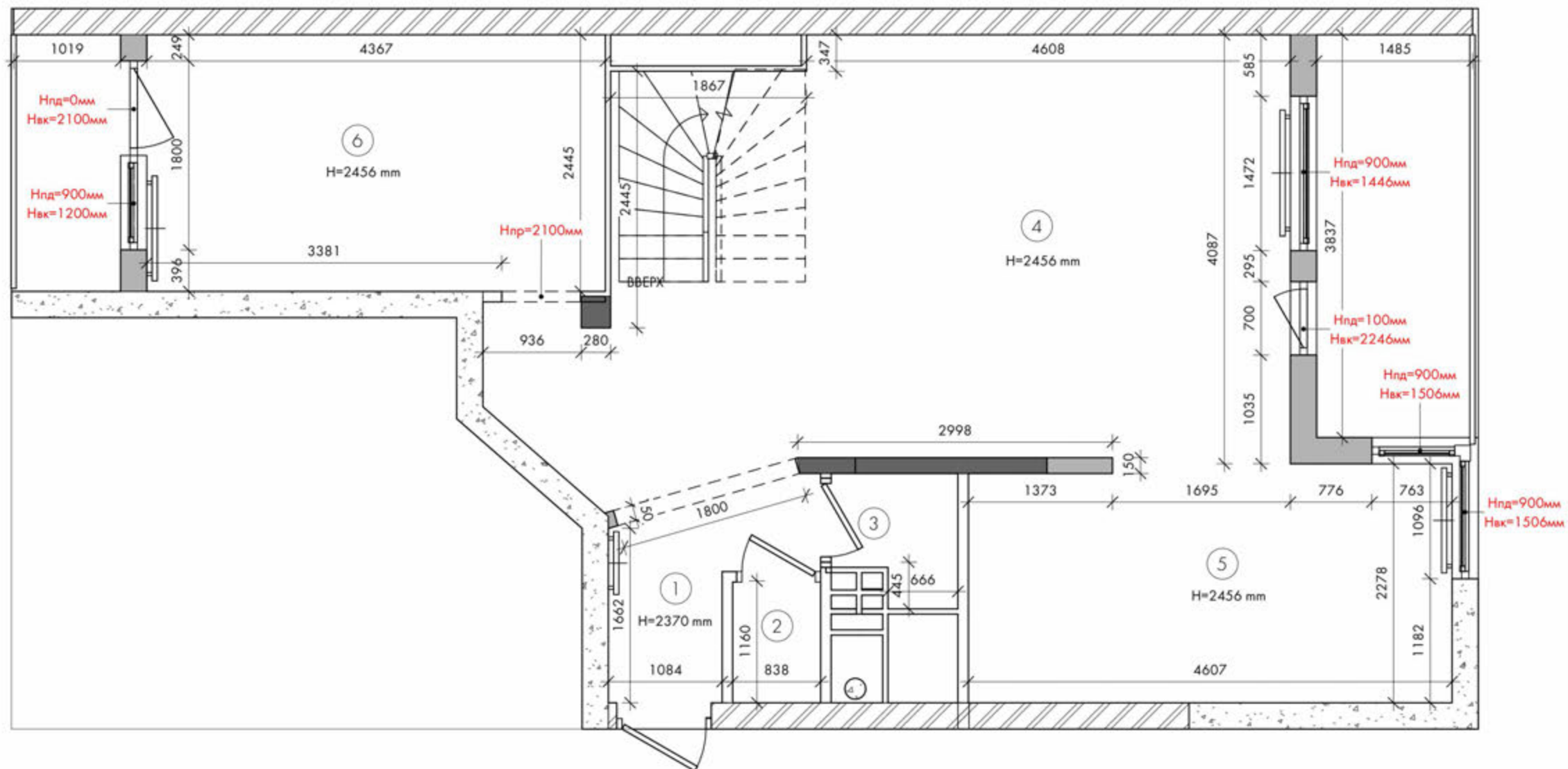
Обмірний план 1 поверх 1 : 50
