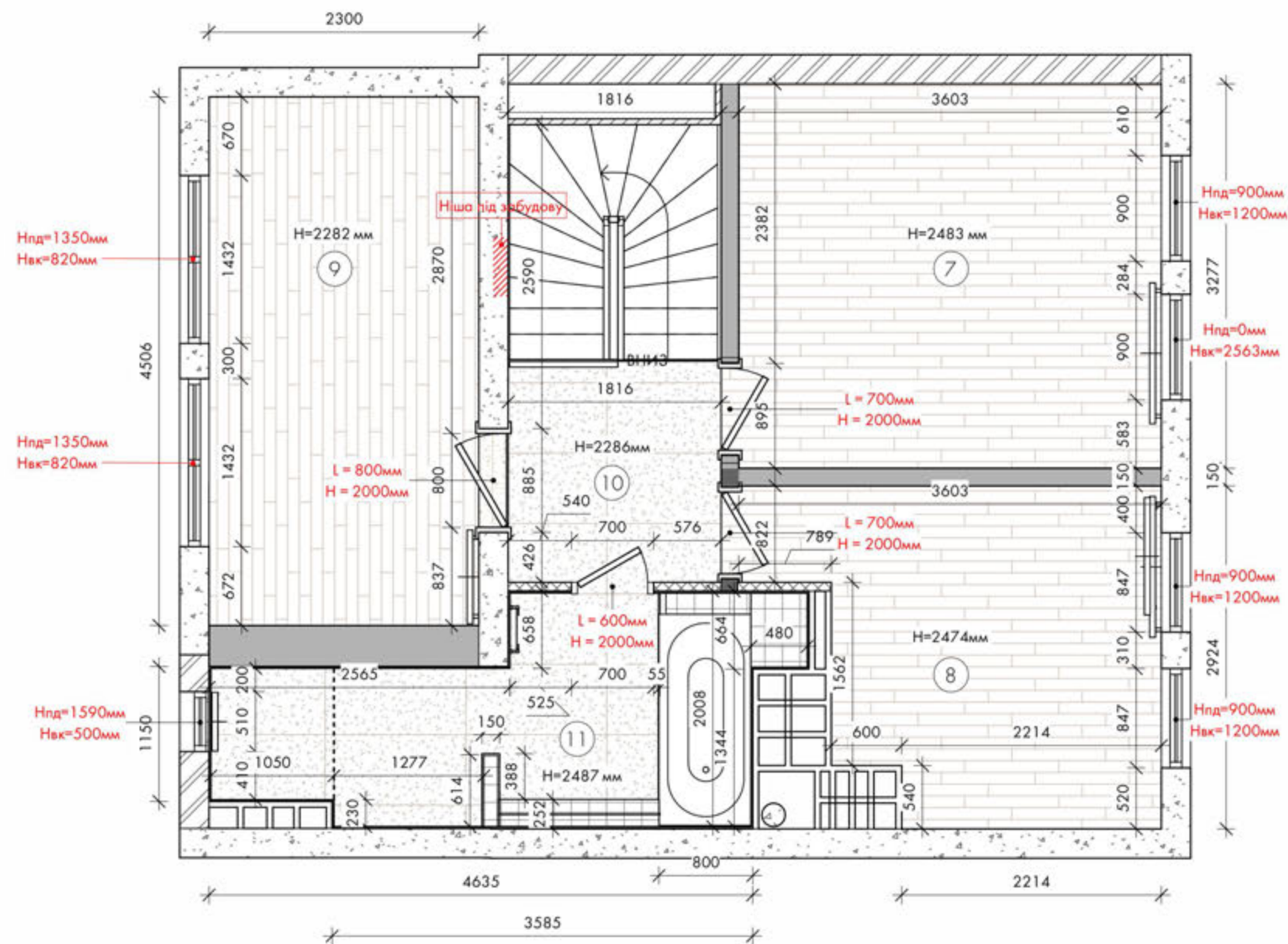
Обмірний план 2 поверху 1:50
