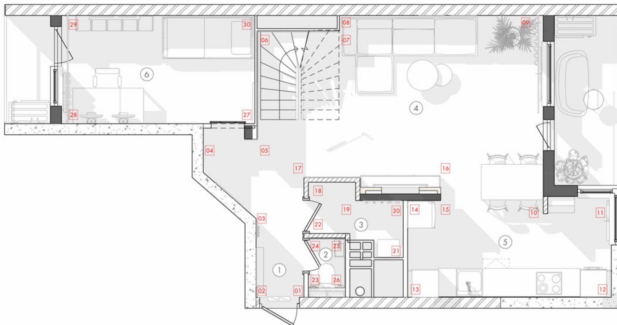
План маркування кутів приміщень 1 : 50
