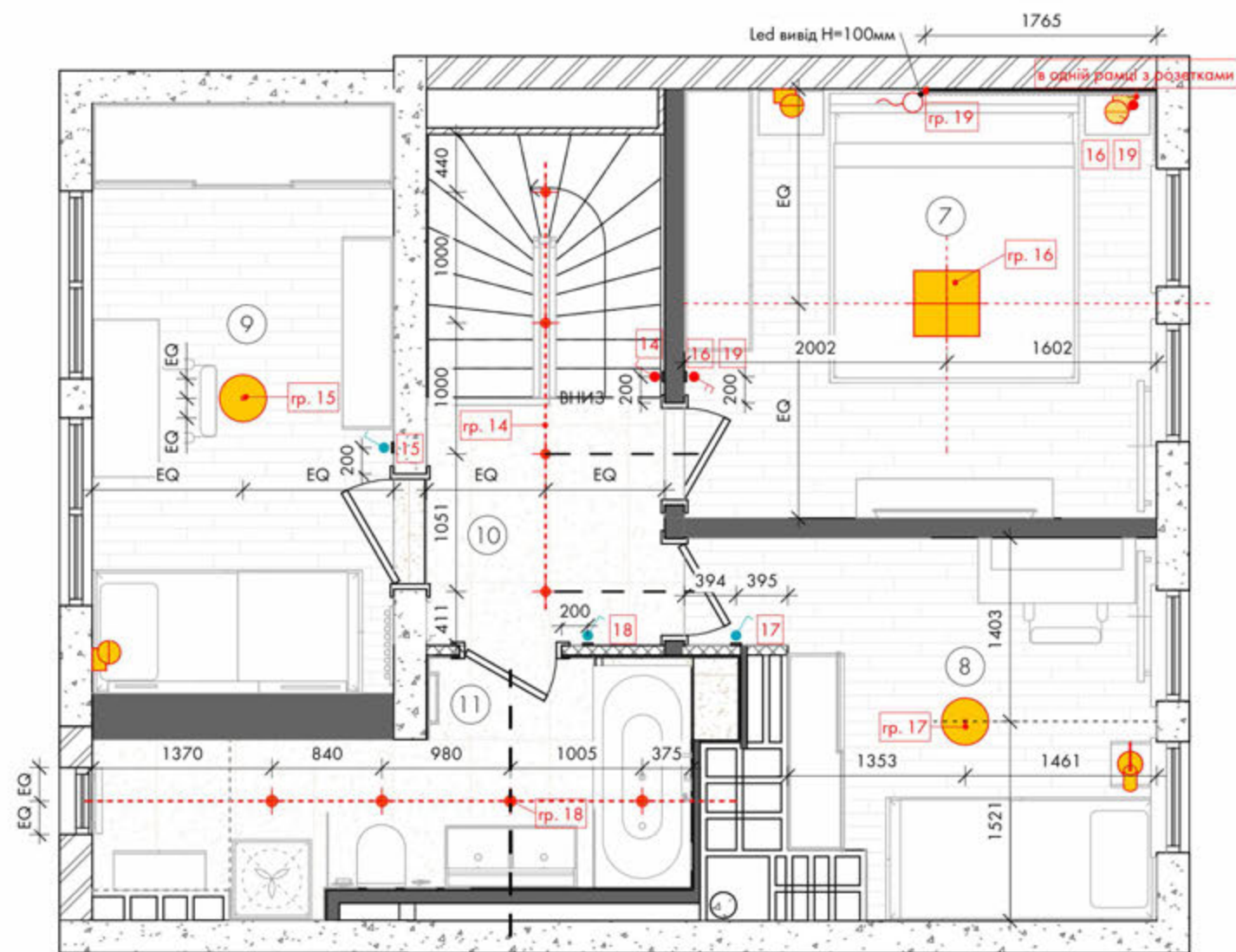
План розміщення освітлювальних приладів 2 поверх
