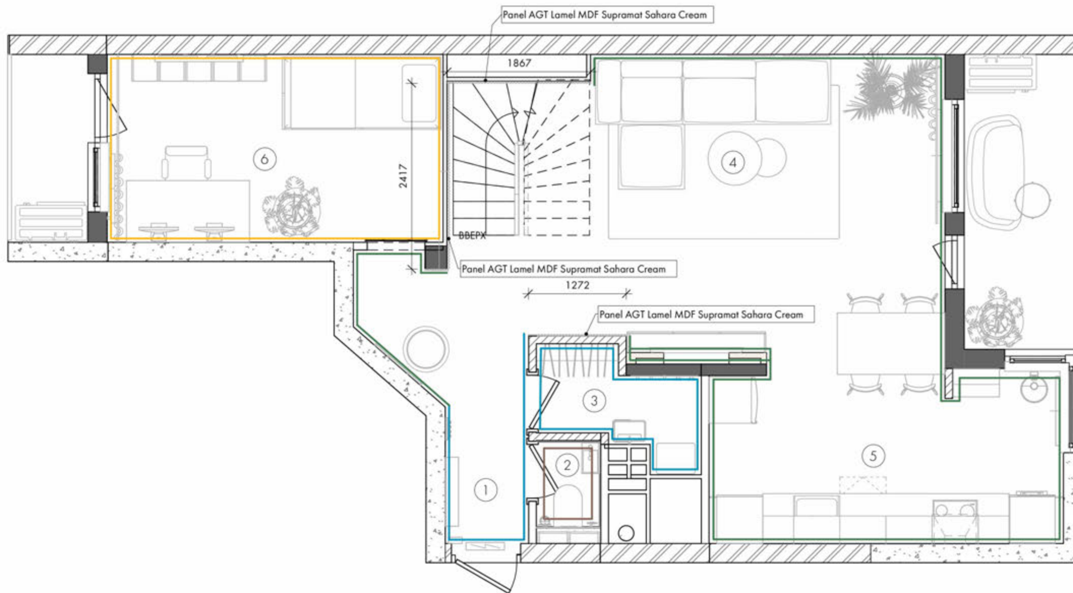
План оздоблювальних матеріалів стін 1 : 50
