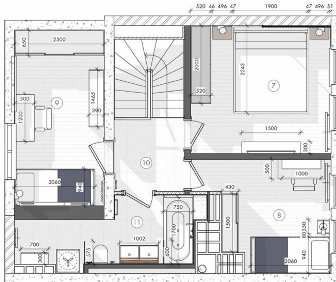
План меблів 2 поверх
