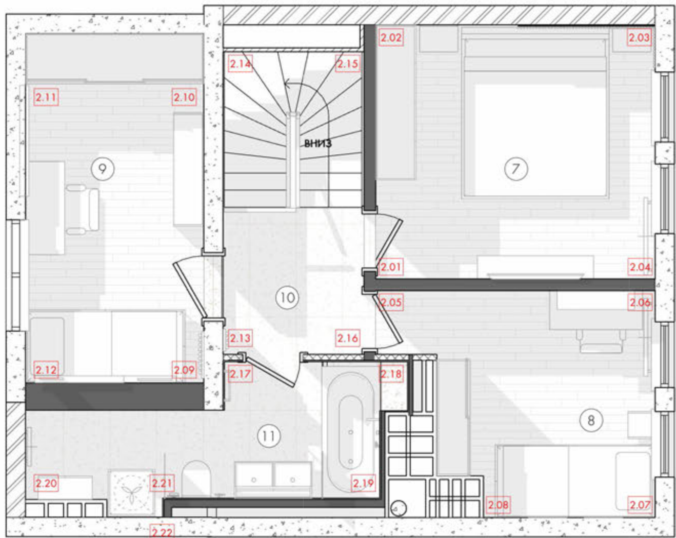
План маркування кутів приміщень 2 поверх
