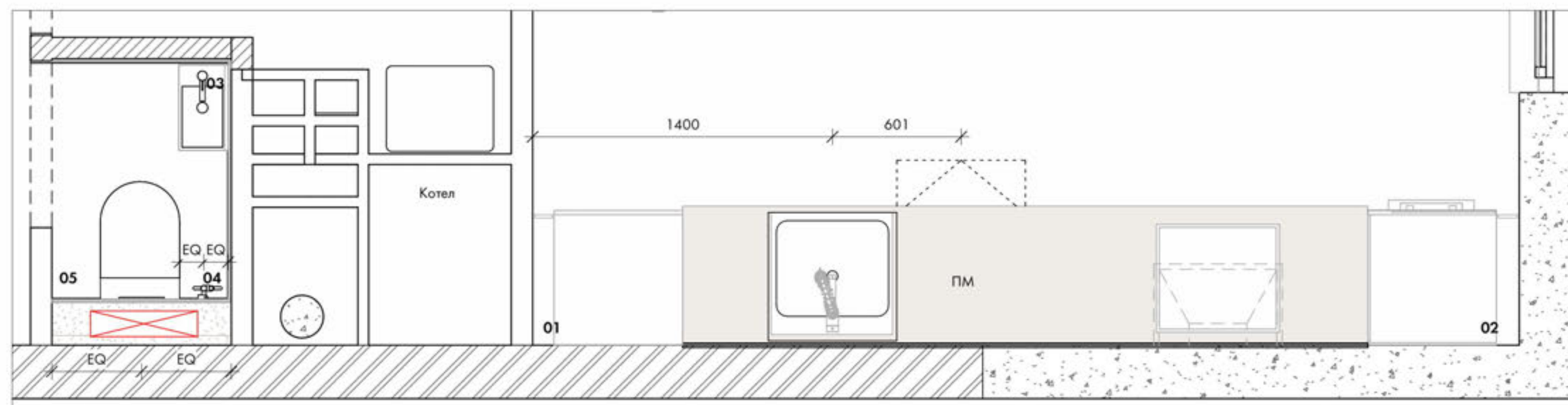
План сантехнічних виводів 1 : 25
