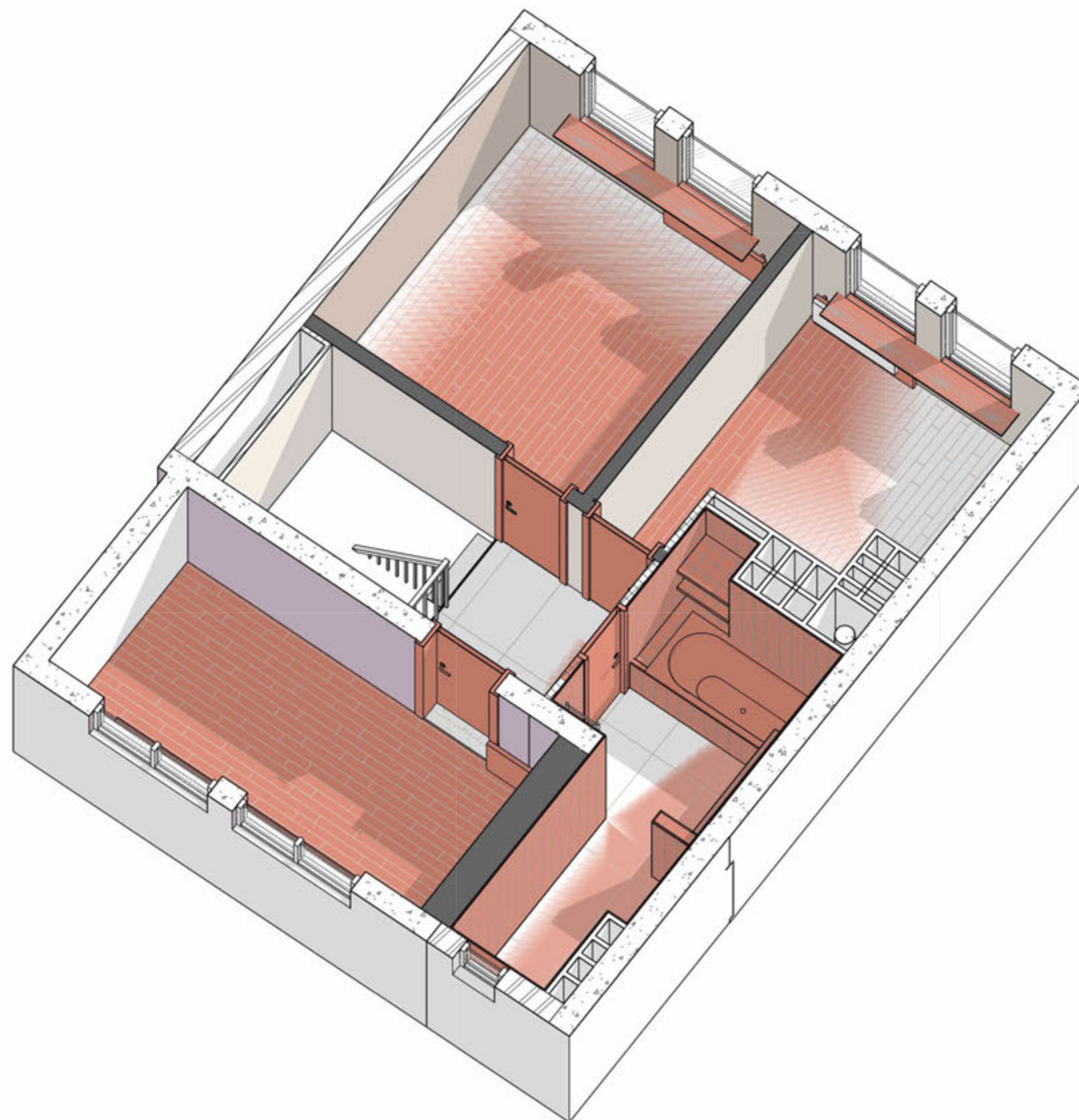
3D демонтаж 2 поверх
