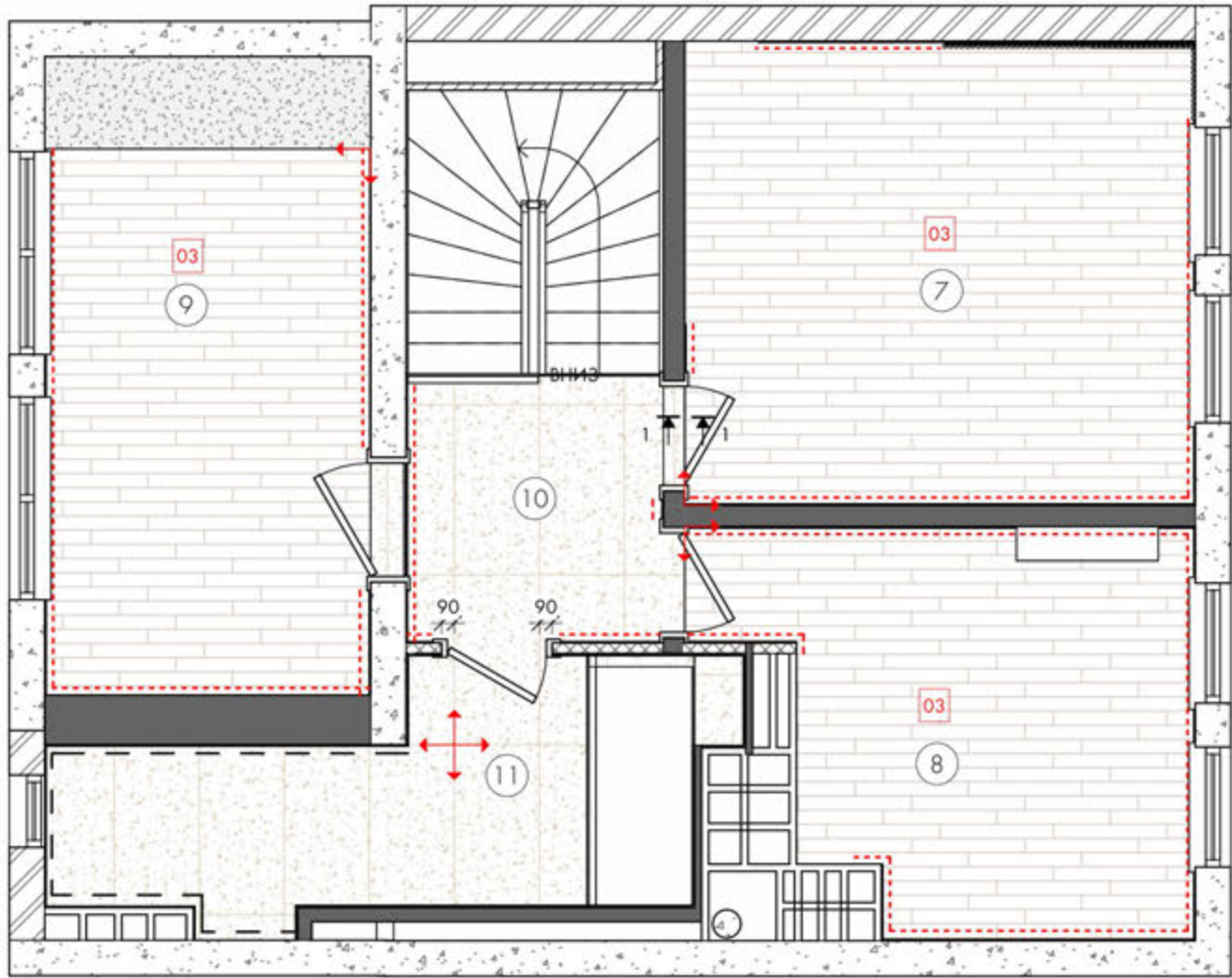
План підлог 2 поверха 1 : 50
