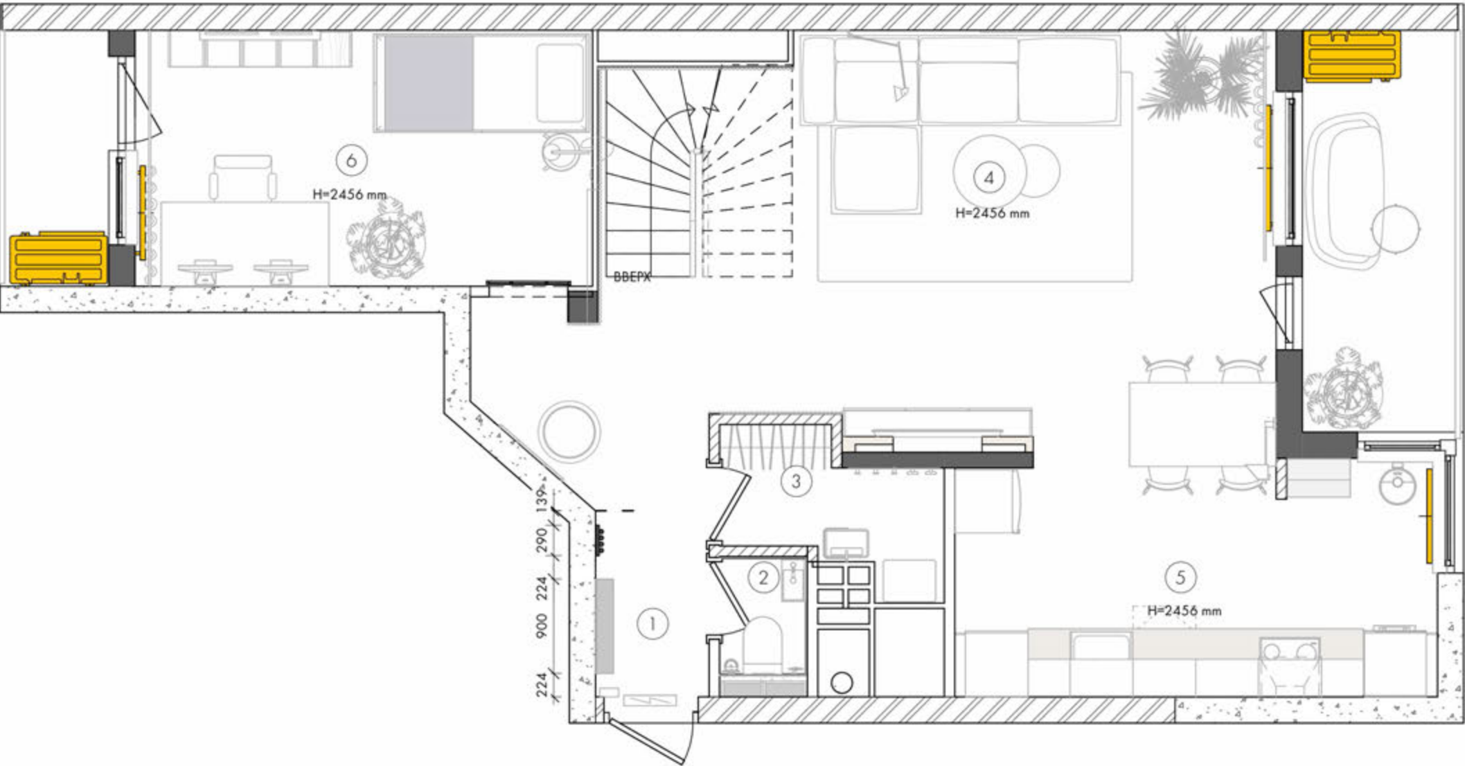
План опалення 1 : 50
