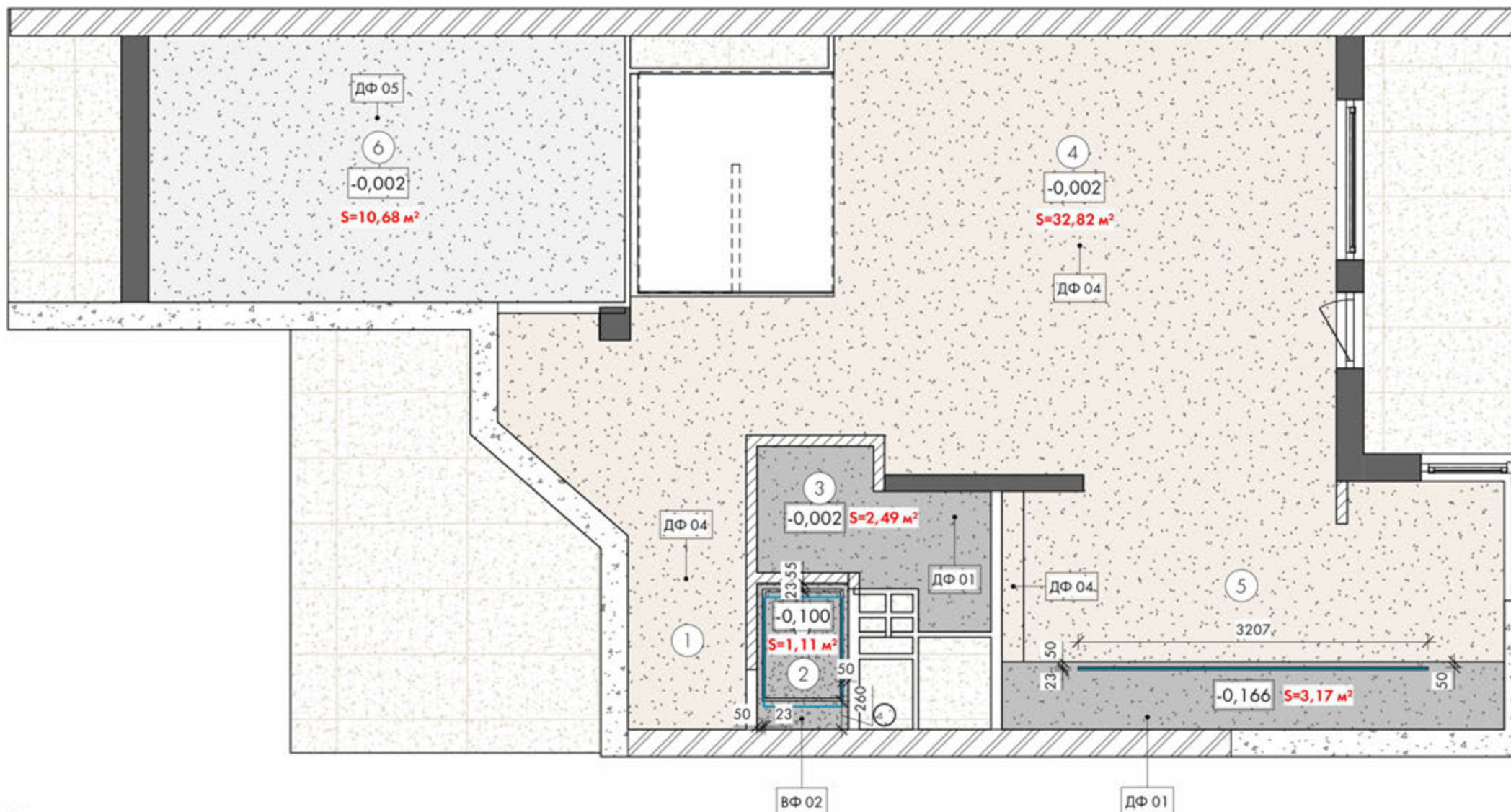
План стель 1 : 50
