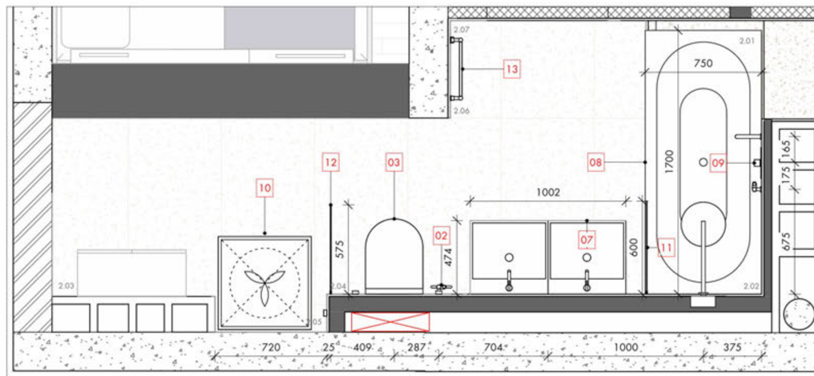
План сантехнічних виводів 2 поверх 1 : 25
