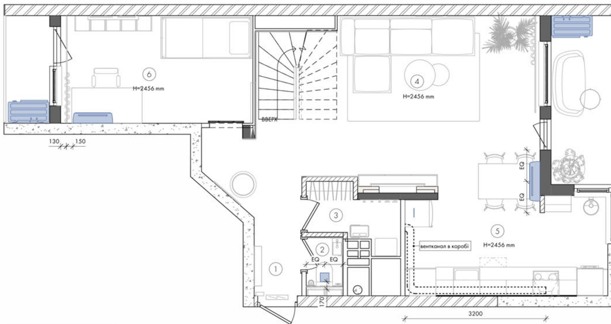
План вентиляції та кондиціонування
