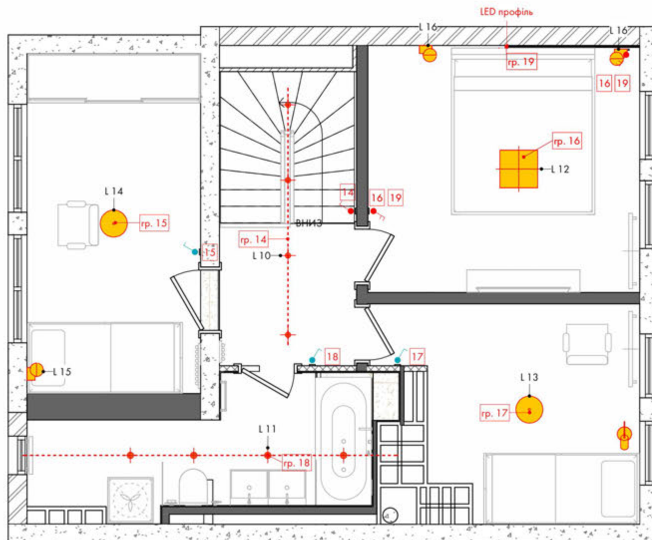
План груп світла та вимикачів 2 поверх 1 : 50
