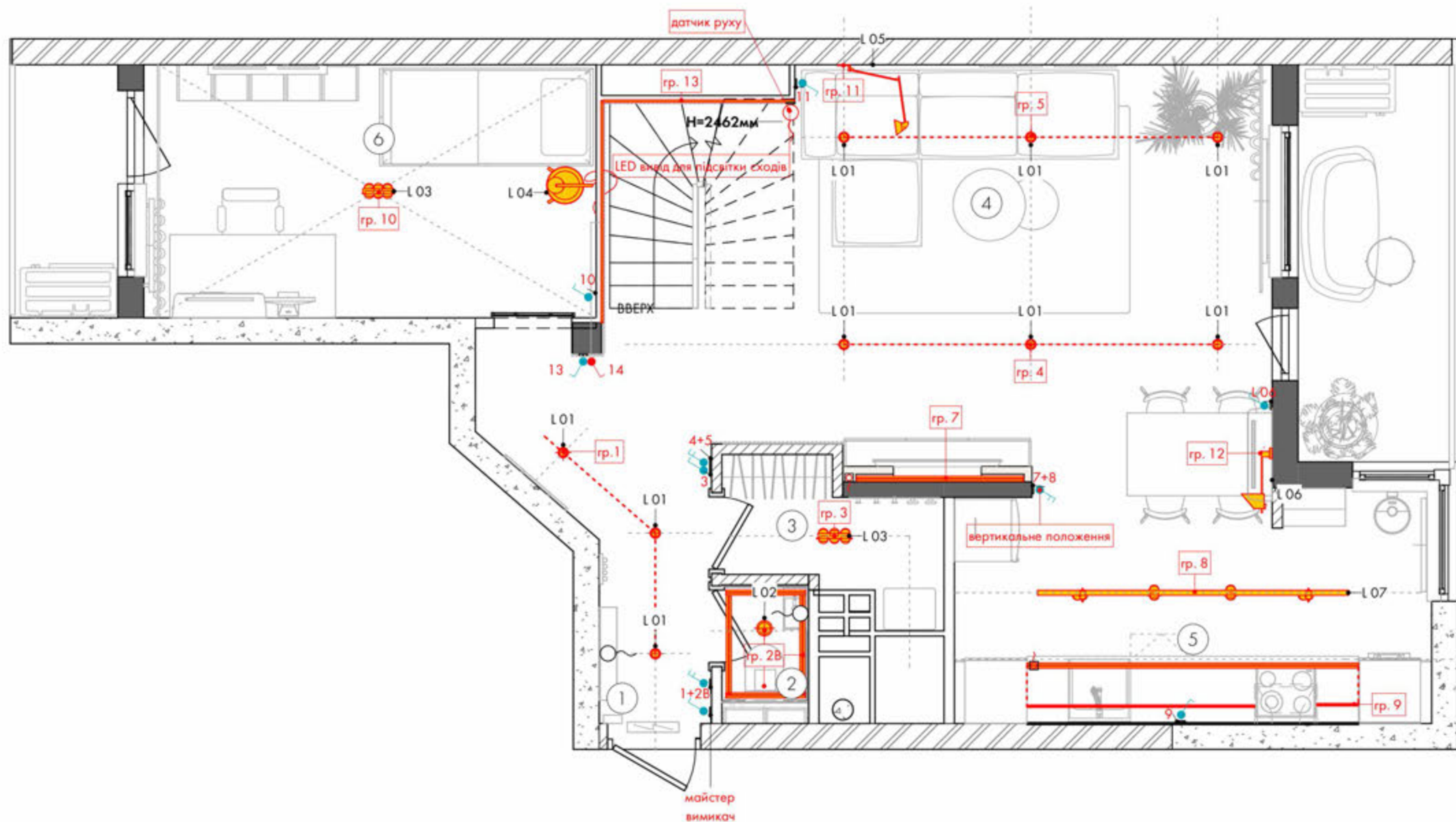
План груп світла та вимикачів 1 : 50
