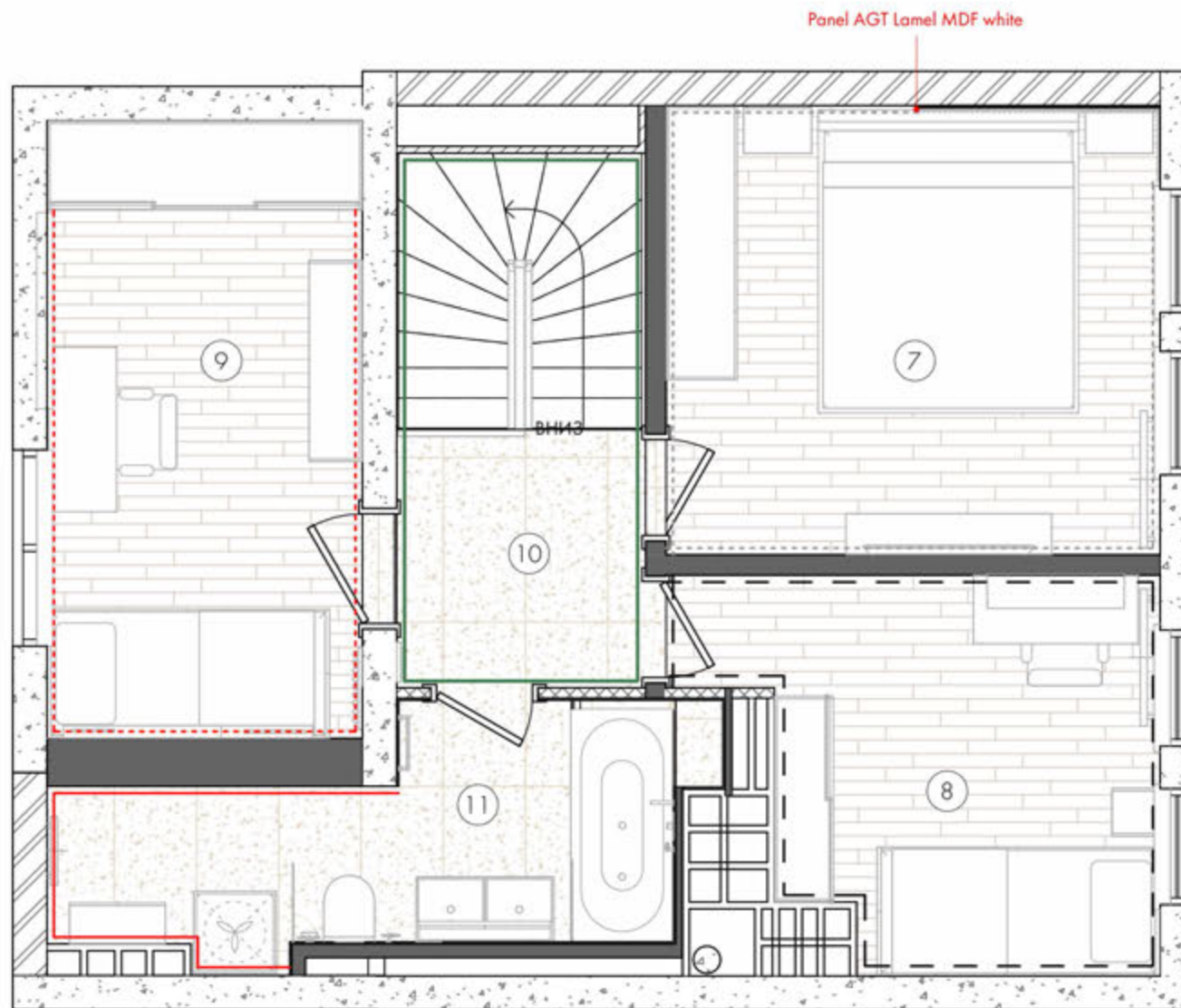
План оздоблювальних матеріалів стін 2 поверх
